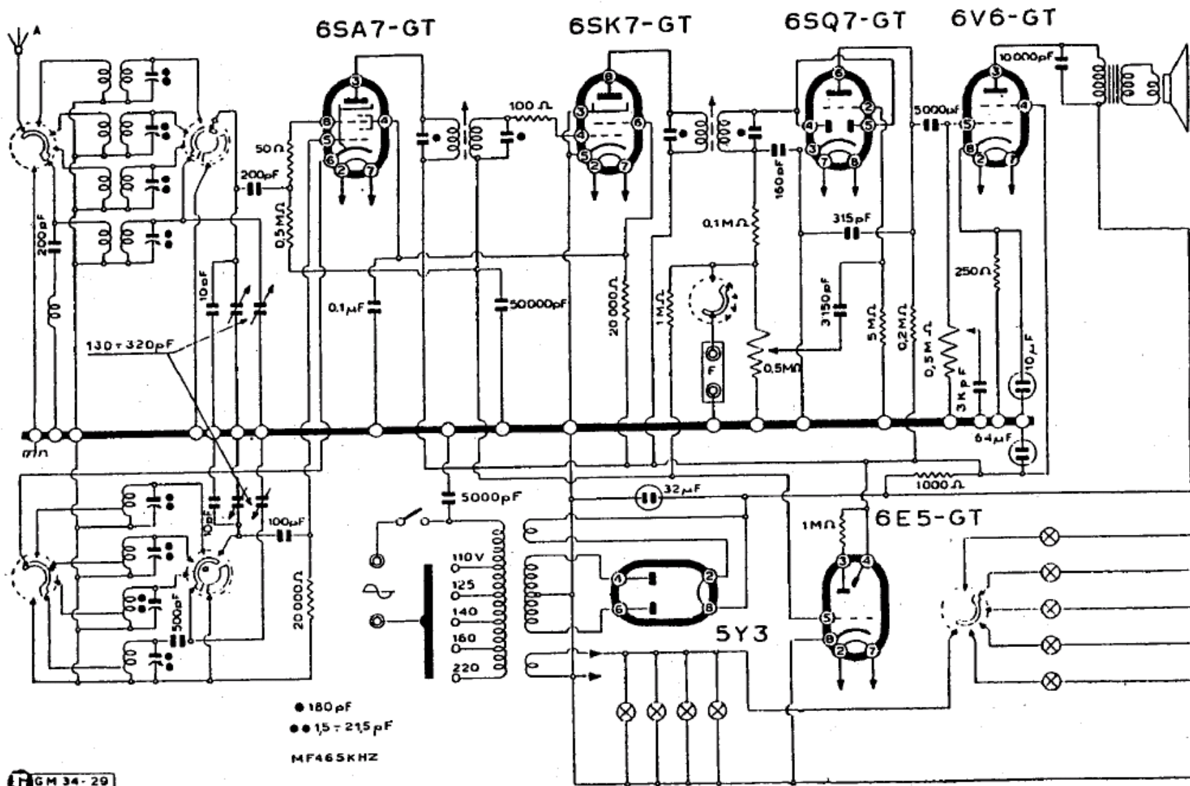
RADIO SUPERLA - Modd. R50/B - R50/C (Il mod. R50C è privo di occhio magico)
